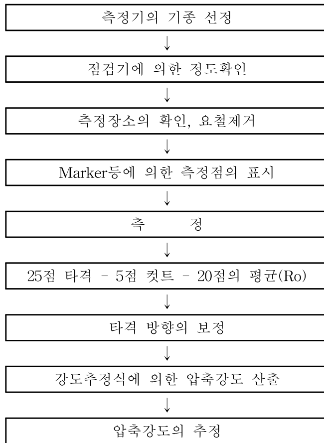
<그림 2.4.1> 반발경도법에 의한 압축강도 추정도
