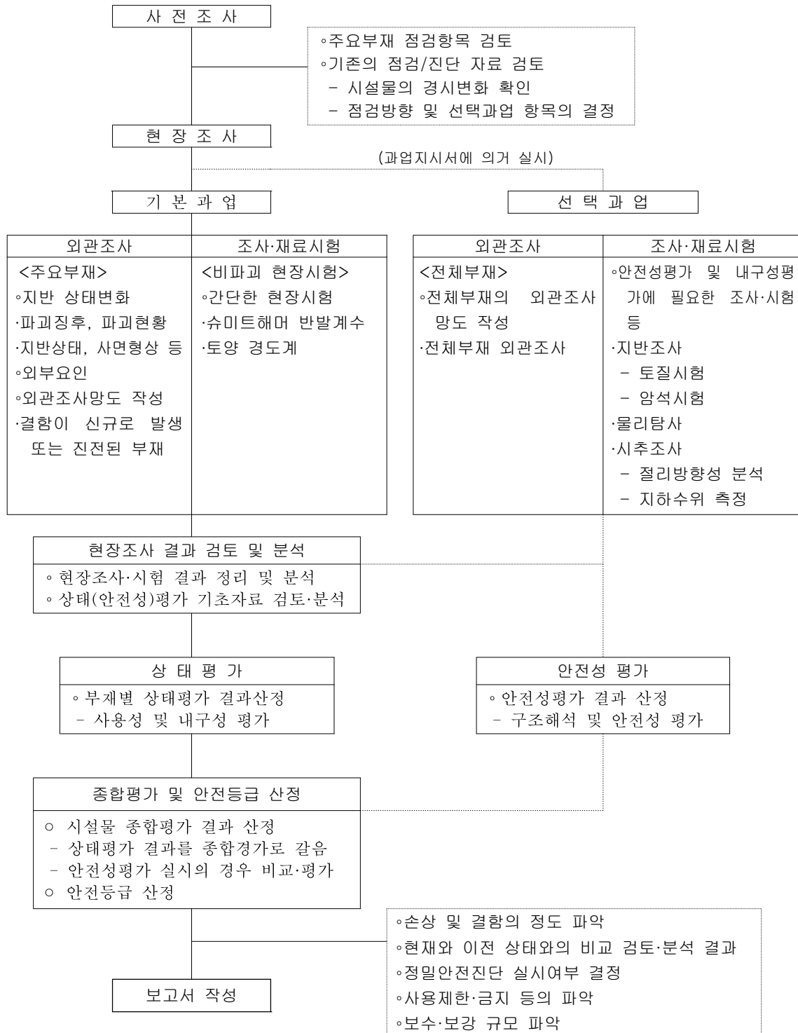
<그림 1.4.1> 절토사면 정밀점검 업무흐름도
